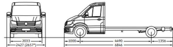
Crafter 35 Chassis lang med enkeltkabine
